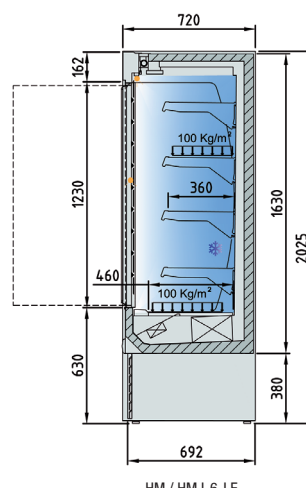
HM / HM I-6-LE
