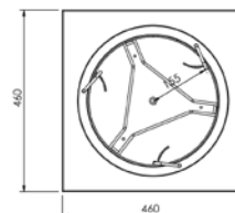
MEDIDAS DISPENSADOR DE PLATOS
