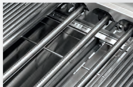
Quemadores Burners
